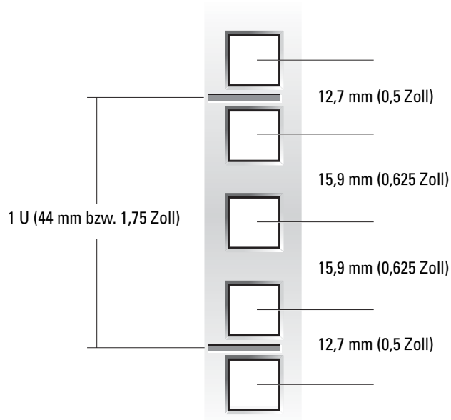
Abbildung 3-3. Eine Rack-Einheit
